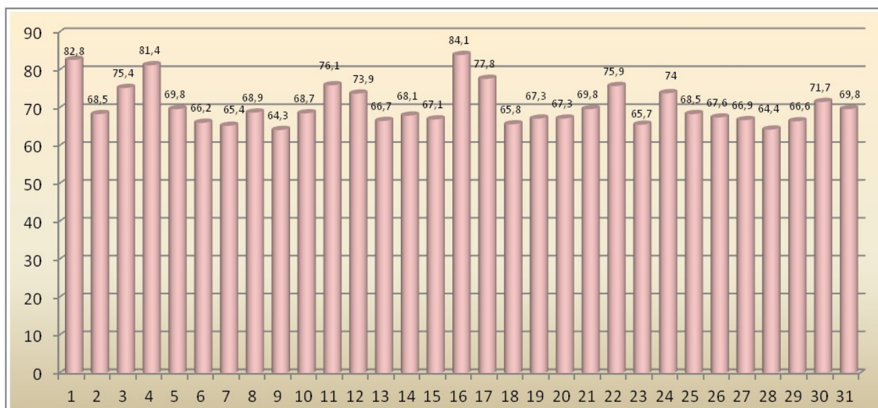
5 pav. Maksimalaus triukšmo pasiskirstymas matavimo vietose dienos metu (7-19val.). Ribinis dydis 70 dBA.
