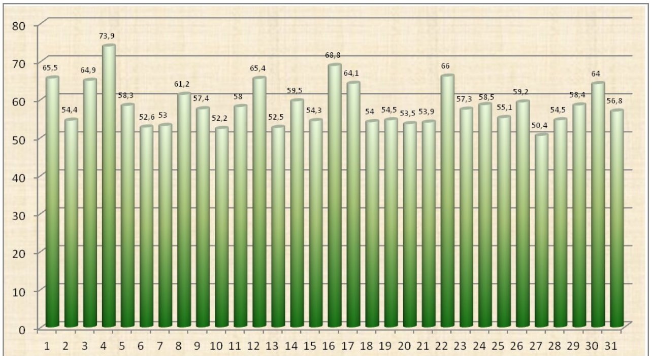
6 pav. Ekvivalentinio triukšmo pasiskirstymas matavimo vietose dienos metu (7-19 val.). Ribinis dydis 65 dBA.
